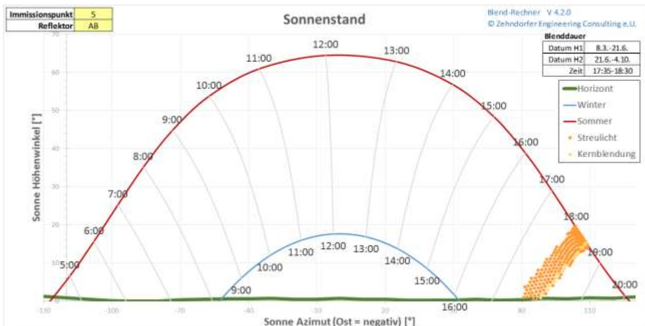
Abbildung 10 Sonnenwinkel bei Blendung am IP 5
