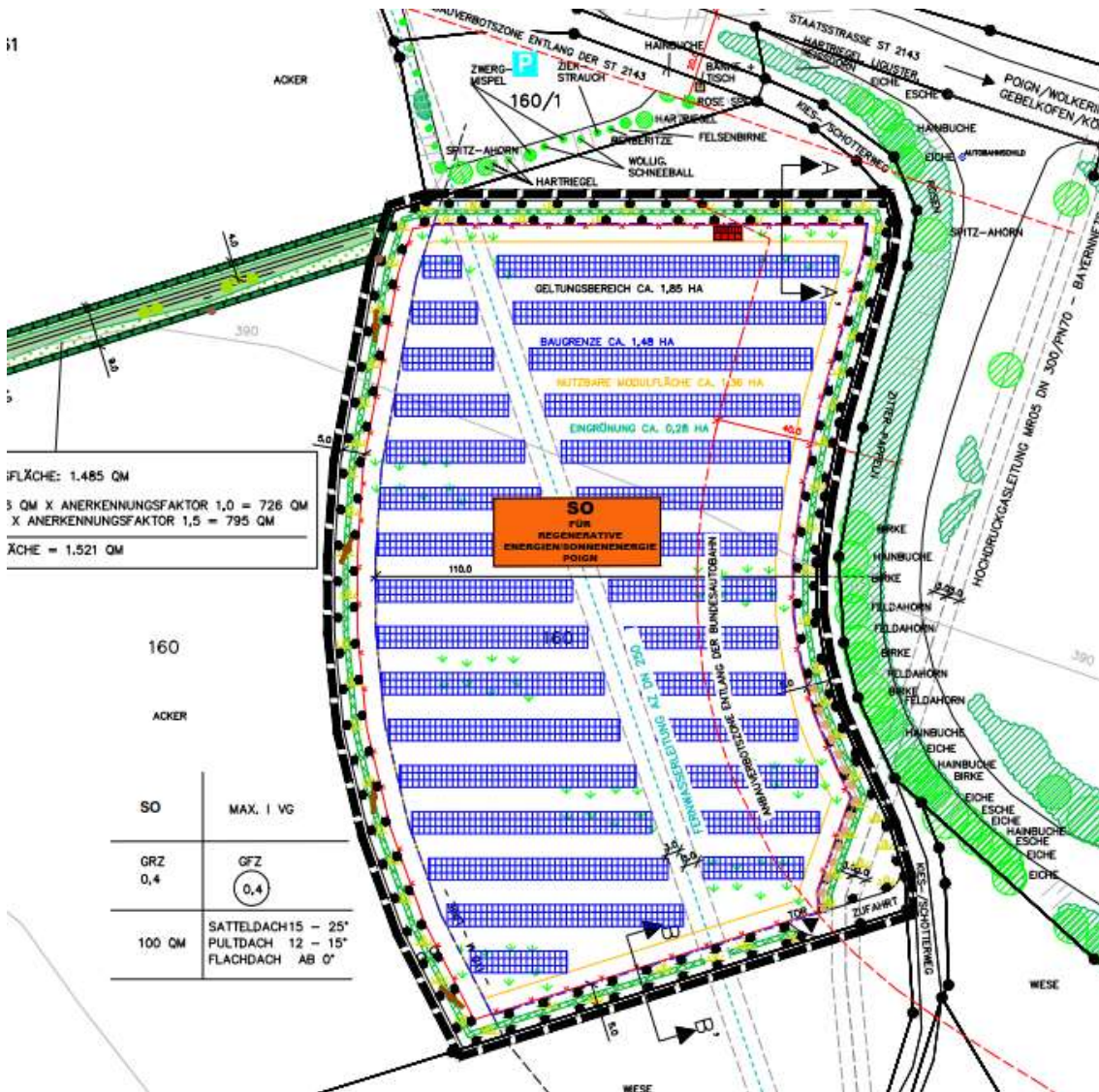
Abbildung 2 Layout der Solar-Anlage
